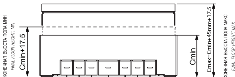
ВЫСОТА СОСТАВА МИН / МАКС ASSEMBLY HEIGHT MIN / MAX
