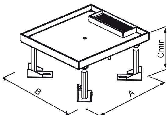
КОНЕЧНАЯ ВЫСОТА ПОЛА MIN FINAL FLOOR HEIGHT: MIN
